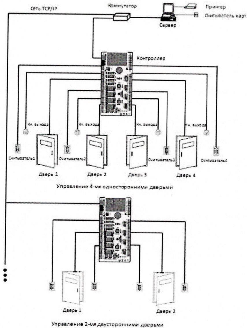
Схема подключения контроллера
