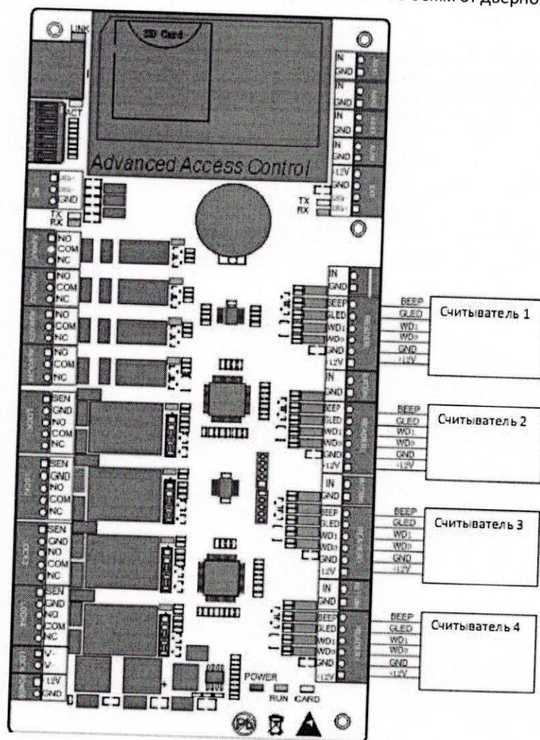
Подключение считывателей к контроллеру C3-400
