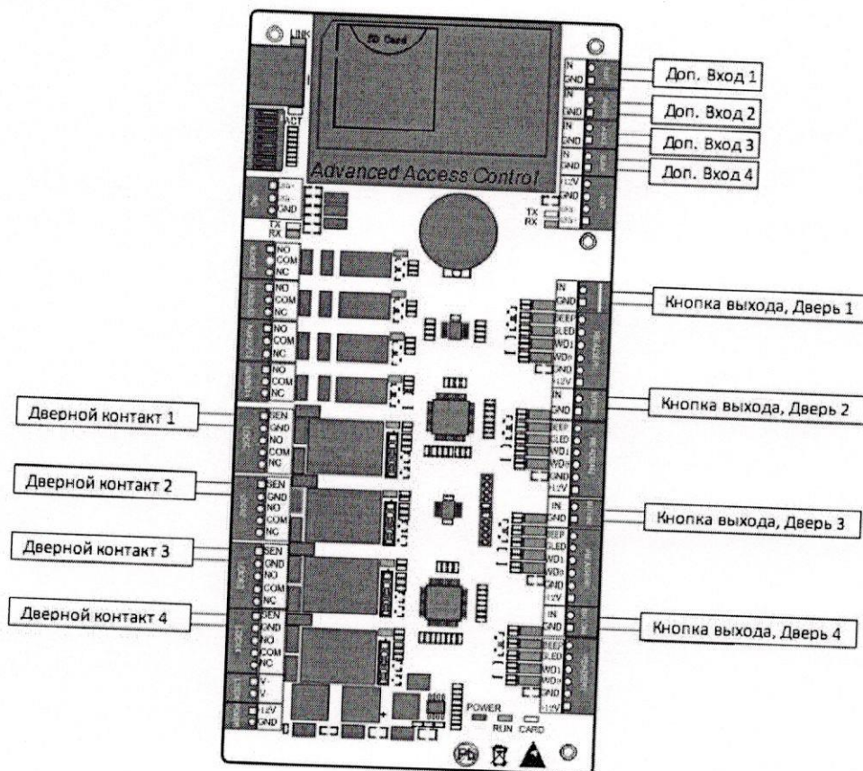
Подключение дверных контактов, кнопок выхода и дополнительных входов контроллера СЗ-400.
