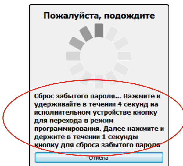
Рисунок 67 – Сброс забытого пароля
